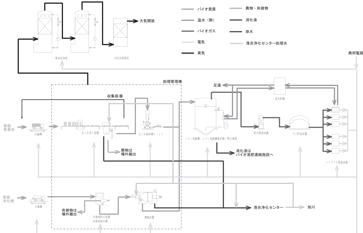
真庭市くらしの循環センターフローシート
