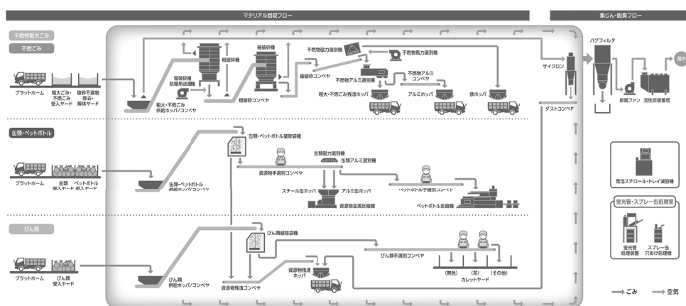
マテリアルリサイクル施設フローシート
