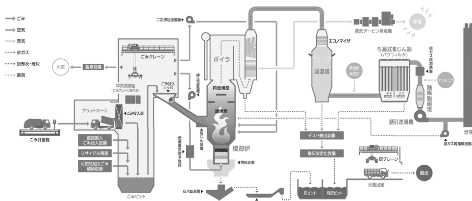
エネルギー回収施設フローシート
