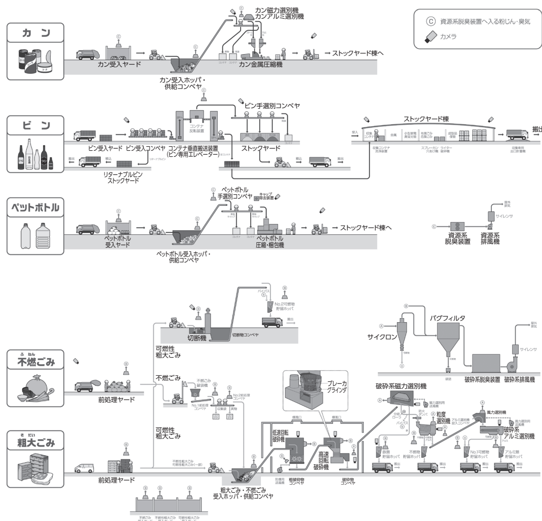
富士山エコパーク再資源化センター フローシート
