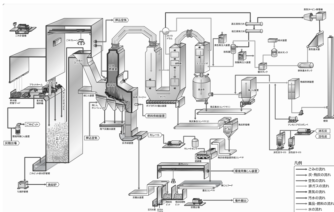
紀の海クリーンセンター フロー図
